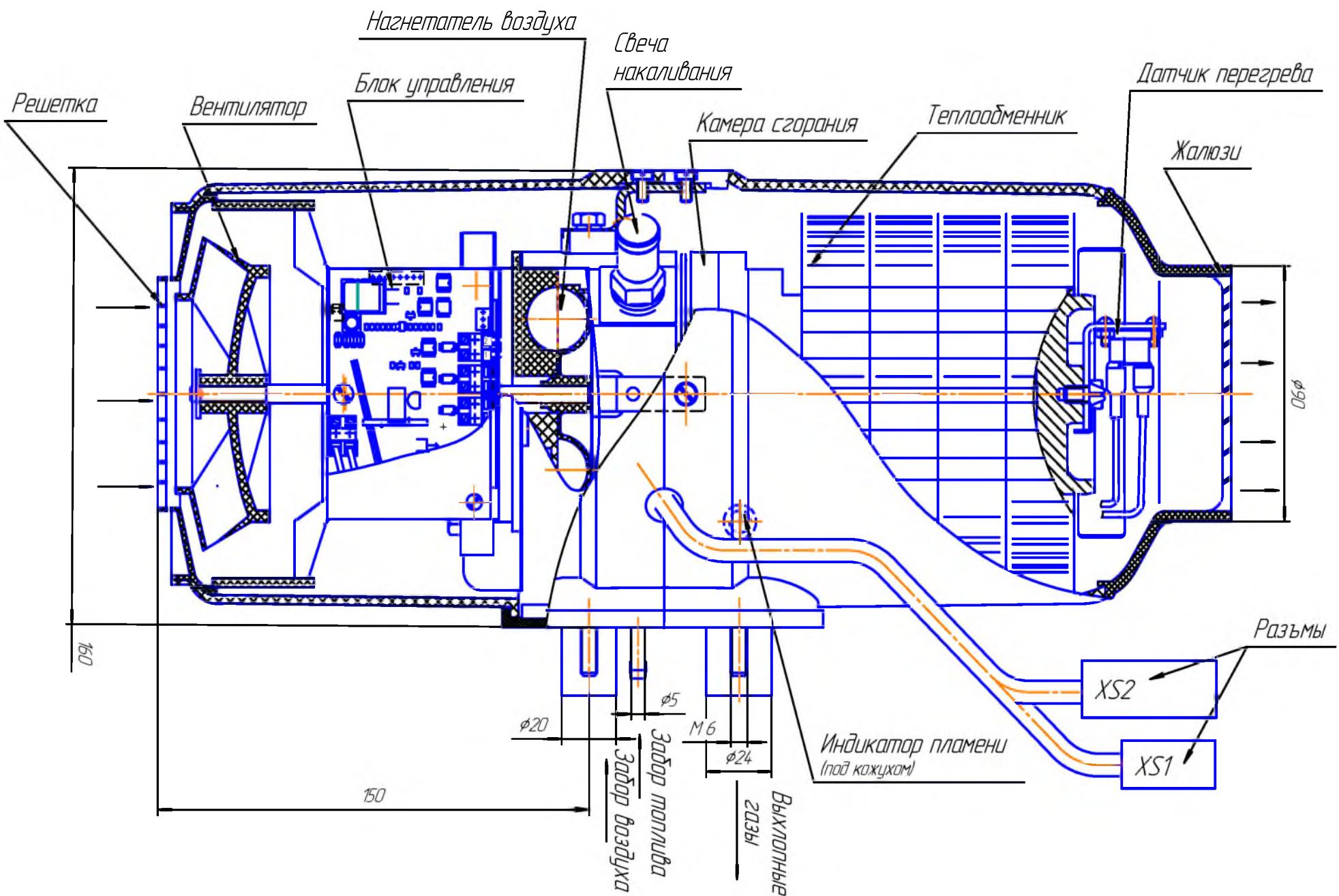
Рис. 4.2 – Основные узлы нагревателя
