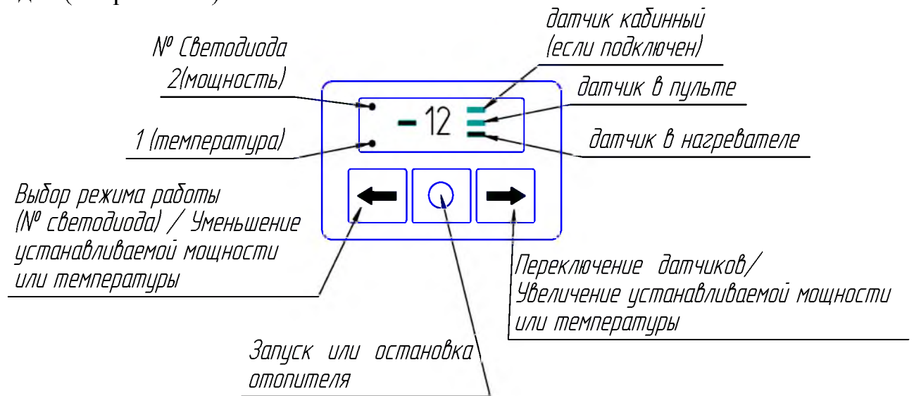
Рис. 6.2.1- Панель пульта
